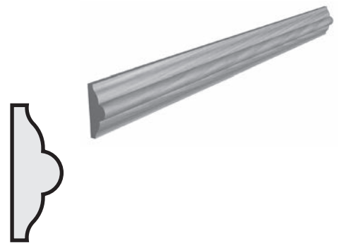
P312 3/8" x 1" ASTRAGAL
